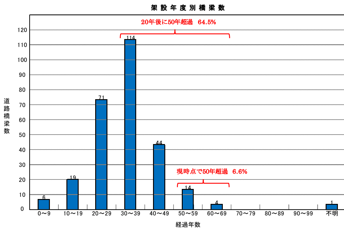
図2-1 吉賀町が管理する道路橋の経過年数ごとの橋梁数
